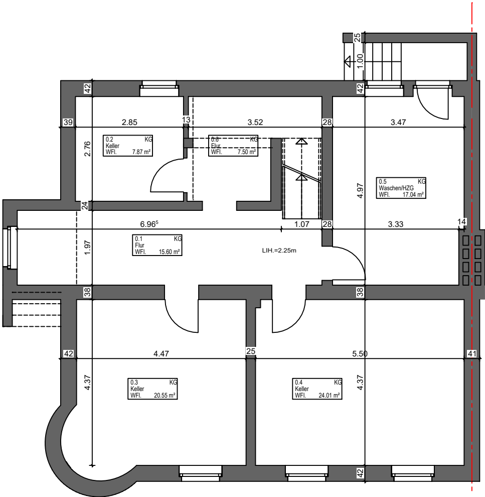
KG 92.57 m²
