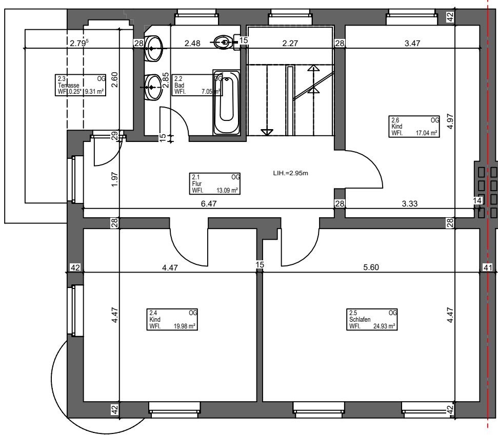
OG 84.41 m²
