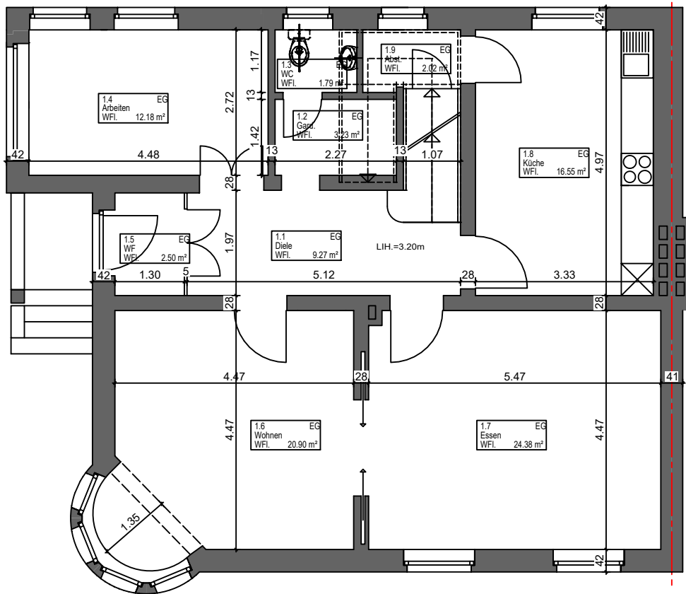
EG 92.82 m²
